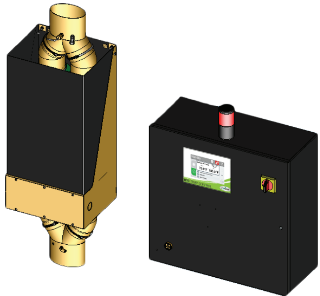
Cada Controlador de Temperatura en Tolva esta equipado con una Caja Calefactora (izquierda) que se conecta directamente a la tolva de secado, y una caja de control de precisión con pantalla táctil. ntrol box with touch screen control.
